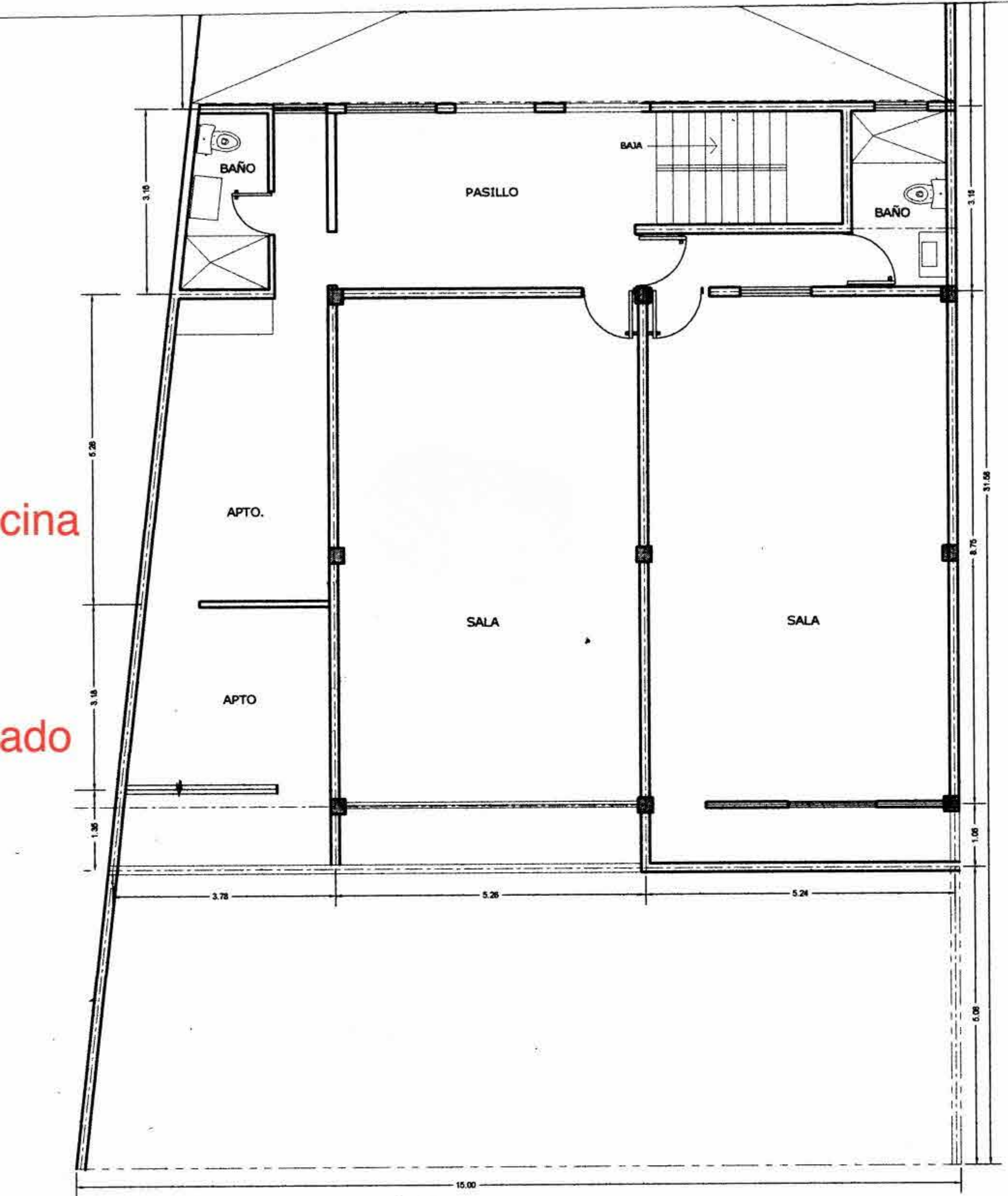
PLANTA 2º NIVEL
